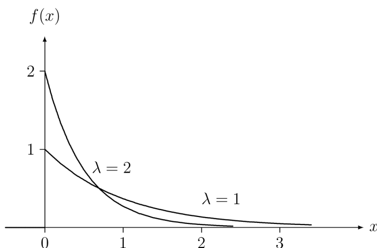
圖 2-17 負指數分配之密度函數
