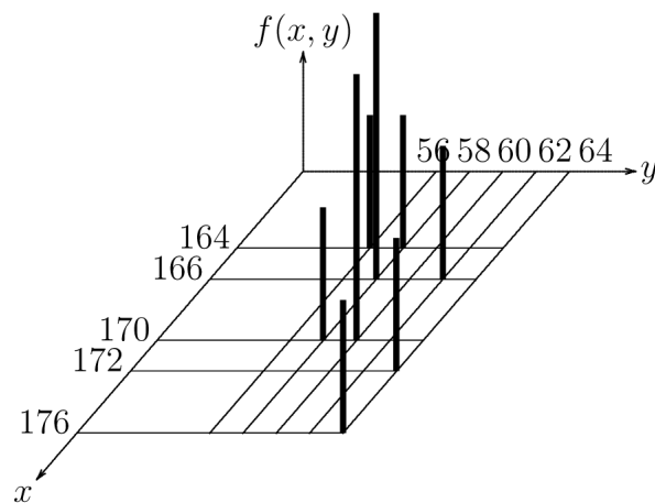
圖 3-4 X 與 Y 之聯合密度函數圖
