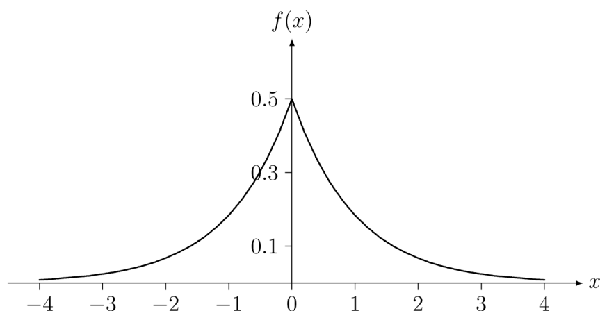
圖 2-22 Laplace 分配之密度函數
