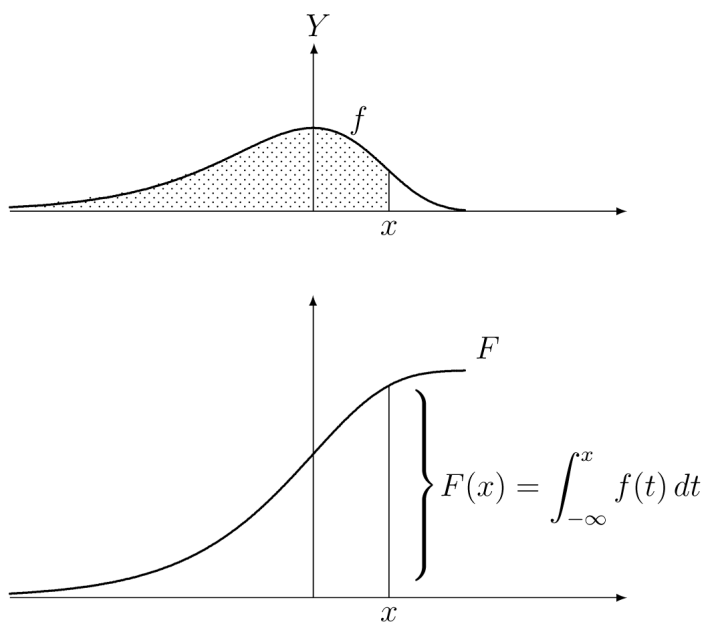
圖 2-8 由密度函數求分配函數
