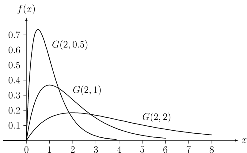
圖 2-15 Gamma 分配之密度函數
