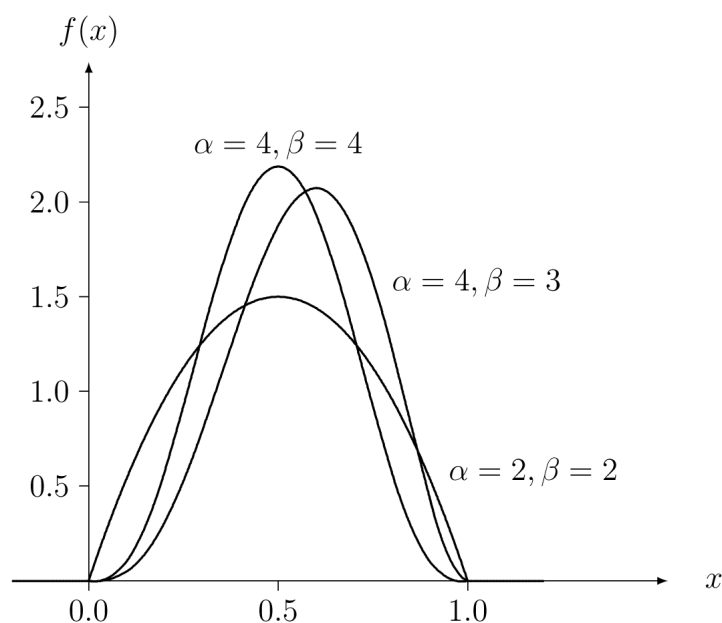
圖 2-19 Beta 分配之密度函數
