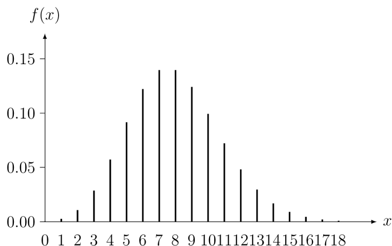
圖 2-10 Poisson 分配 P(8) 之密度函數
