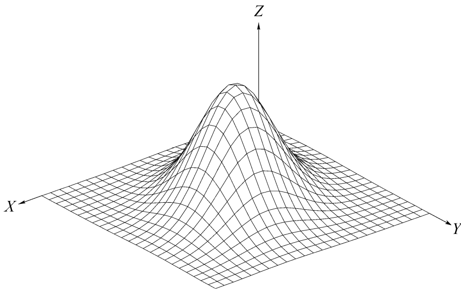
圖 3-1A 二元常態分配之密度函數, \rho = 0.3
